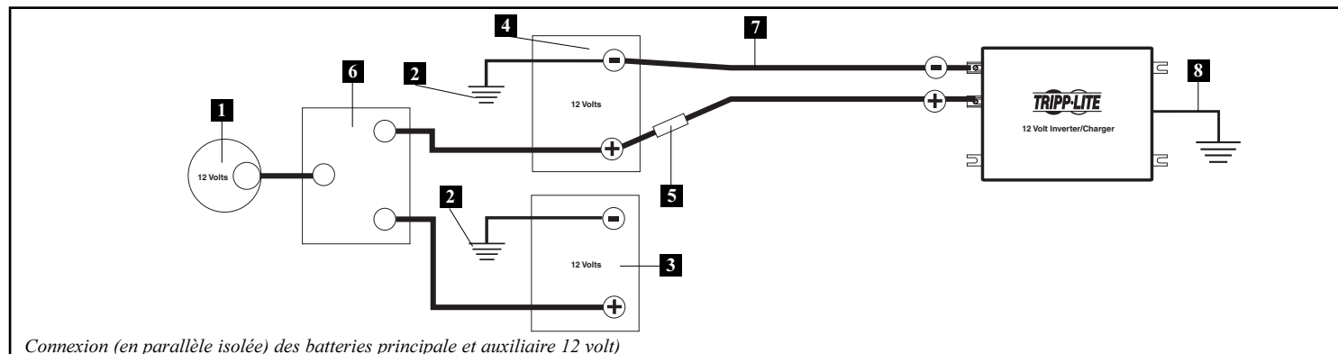
Connexion (en parallèle isolée) des batteries principale et auxiliaire 12 volt
